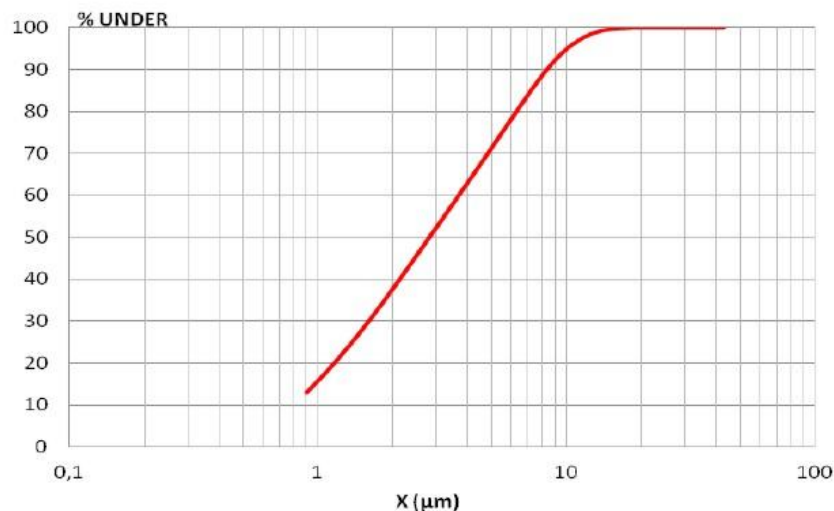
Гранулометрический состав (по SYMPATEC)
