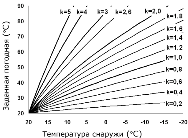
Рис. 5 Кривые нагрева.
