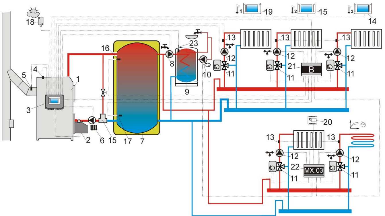
Рис. 11 Схема с тепловым буфером и с 5 смесительными нагревательными контурами 3 , где: 1 – котёл, 2 – горелка, 3 – регулятор, 4 – датчик температуры котла, 5 – датчик температуры продуктов сгорания, 6 – Насос котла, 7 – тепловой буфер, 8 – насос горячего водоснабжения, 9 – резервуар горячего водоснабжения, 10 – циркуляционный насос, 11 – трехходовой клапан с приводом, 12 – насос контура смесителя, 13 – датчик температуры контура смесителя, 14 – комнатная панель ecoSTER200/ecoSTER TOUCH, 15 – комнатная панель ecoSTER200, 16 – верхний датчик температуры буфера, 17 – нижний датчик температуры буфера, 18 – погодный датчик температуры, 19 – комнатная панель ecoSTER200, 20 – стандартный комнатный термостат (замыкательно-размыкательный), 21 – дополнительный модуль В, 22 – дополнительный модуль МХ.03 (модуль С), 23 – датчик температуры горячего водоснабжения СТ4.
