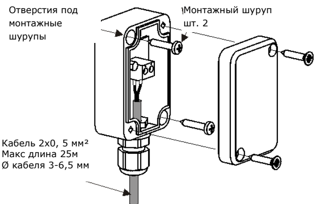
Рис. 16 Подключение датчика погоды СТ4-Р
