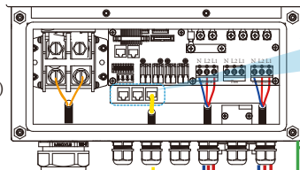
Інвертор №3 (підлеглий)
