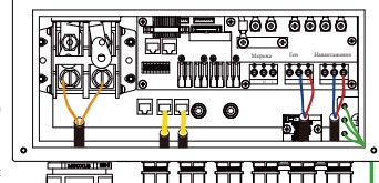
Інвертор №2 (підлеглий)
