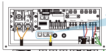
Інвертор №3 (підлеглий)
