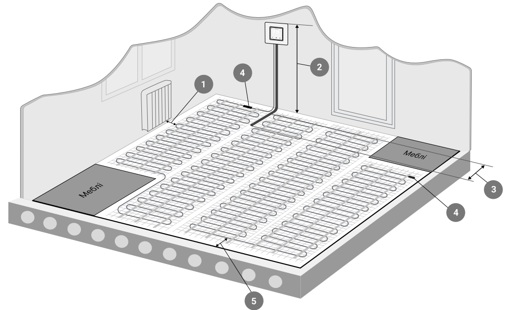
Рис.2 Приклад укладки нагрівального мату
