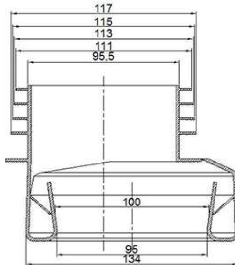
SEZIONE A-A SECTION A-A
