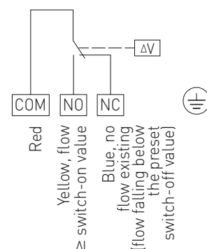
Схема подключения
