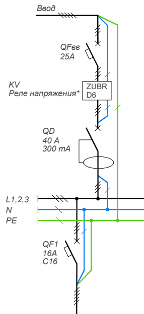
Схема 1. Вариант подключения УЗО, автоматического выключателя с транзитом нуля через устройство к трехфазной нагрузке
