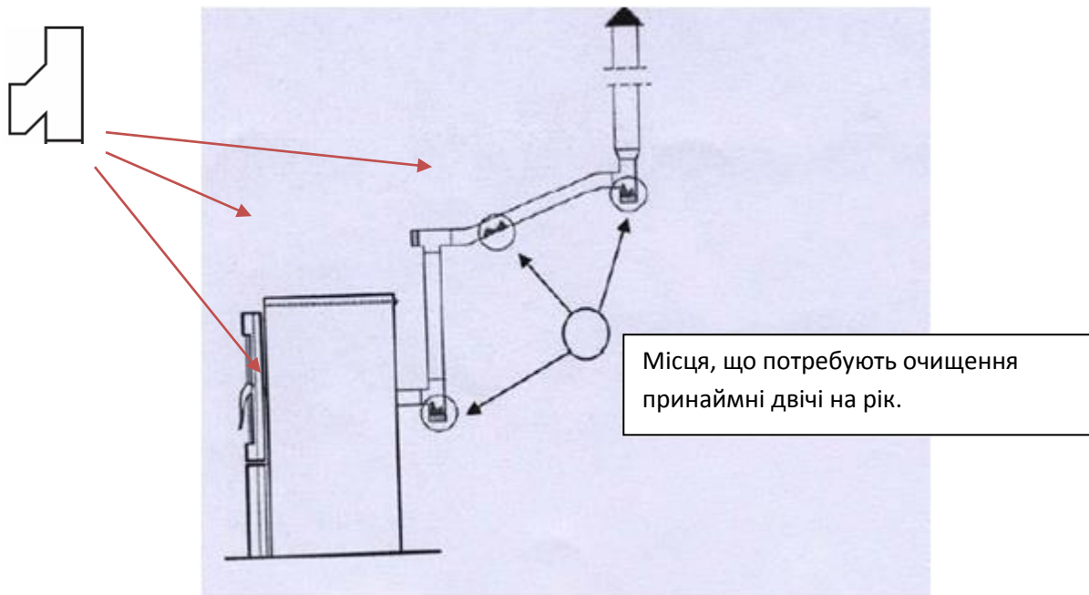
Рис. 17 Місця, що потребують очищення принаймні двічі на рік.
