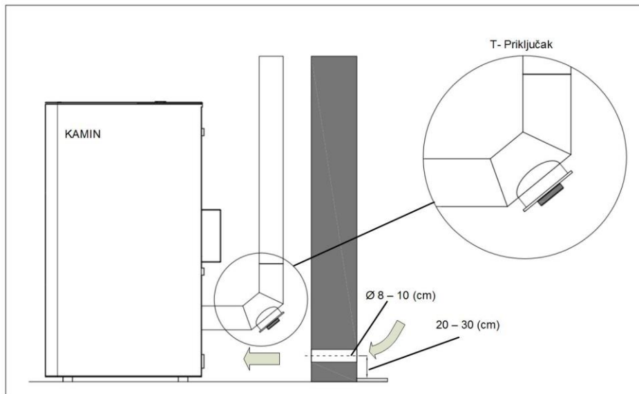
Рисунок 8: Мінімальні зазори для встановлення вентиляційних решіток.
