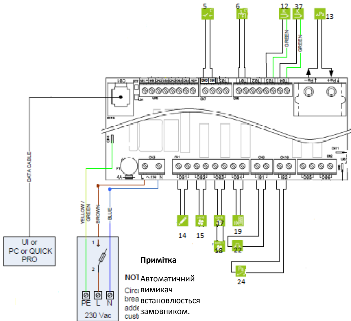
Рисунок 30: Електрична схема
