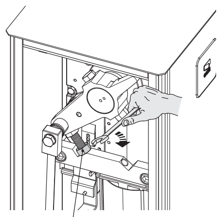
Контргайка
