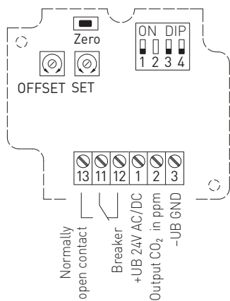
Схема подключения KC02-W
