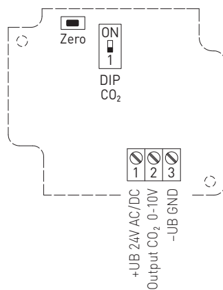
Схема подключения KC02-SD
