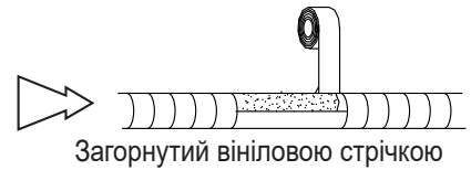
Теплоізоляція труби
