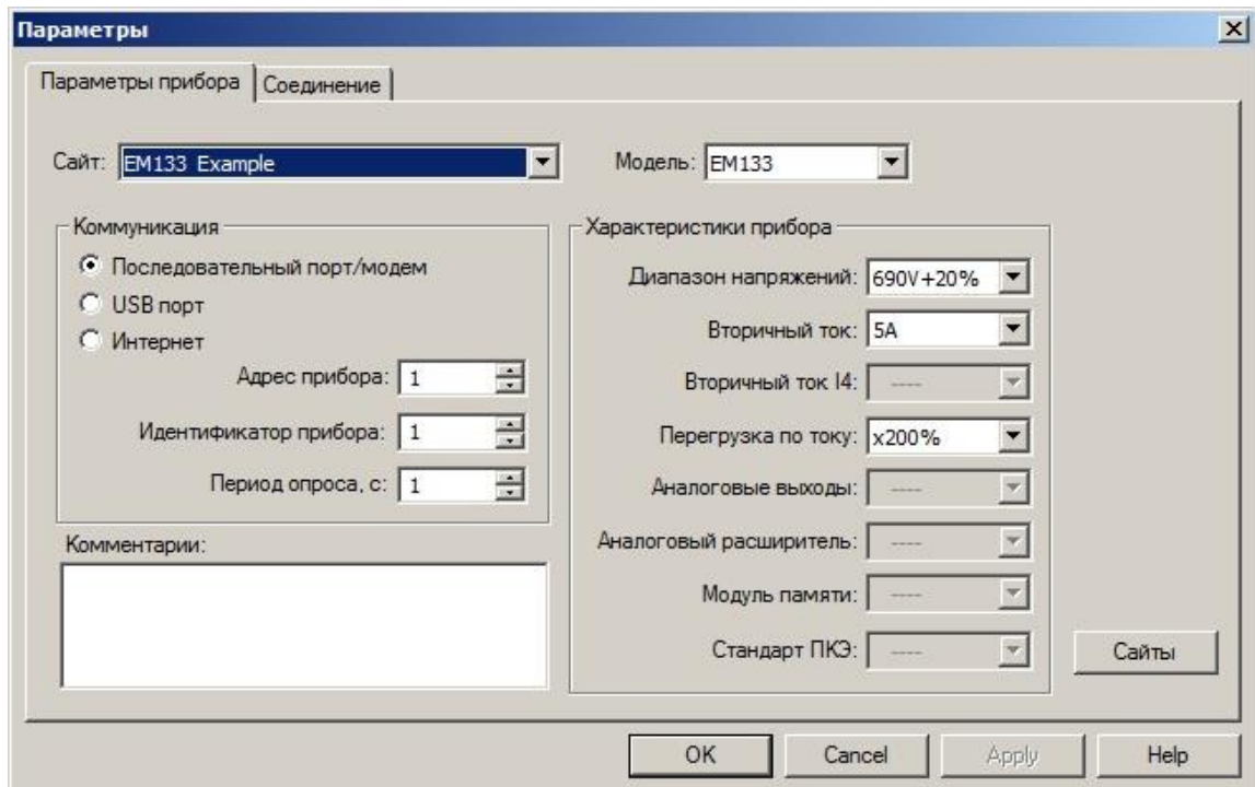
Рисунок 4-1 Диалоговое окно Configuration (Параметры) – Залка Instrument Setup (Параметры прибора)
