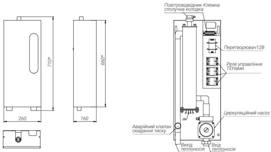
Мал. 1 - Електричний котел. Габаритні розміри.
