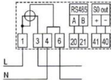
Рис. 1. Схема підключення лічильника
