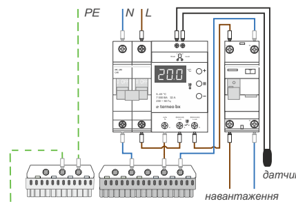
Схема 1. Схема підключення терморегулятора та автоматичного вимикача і ПЗВ
