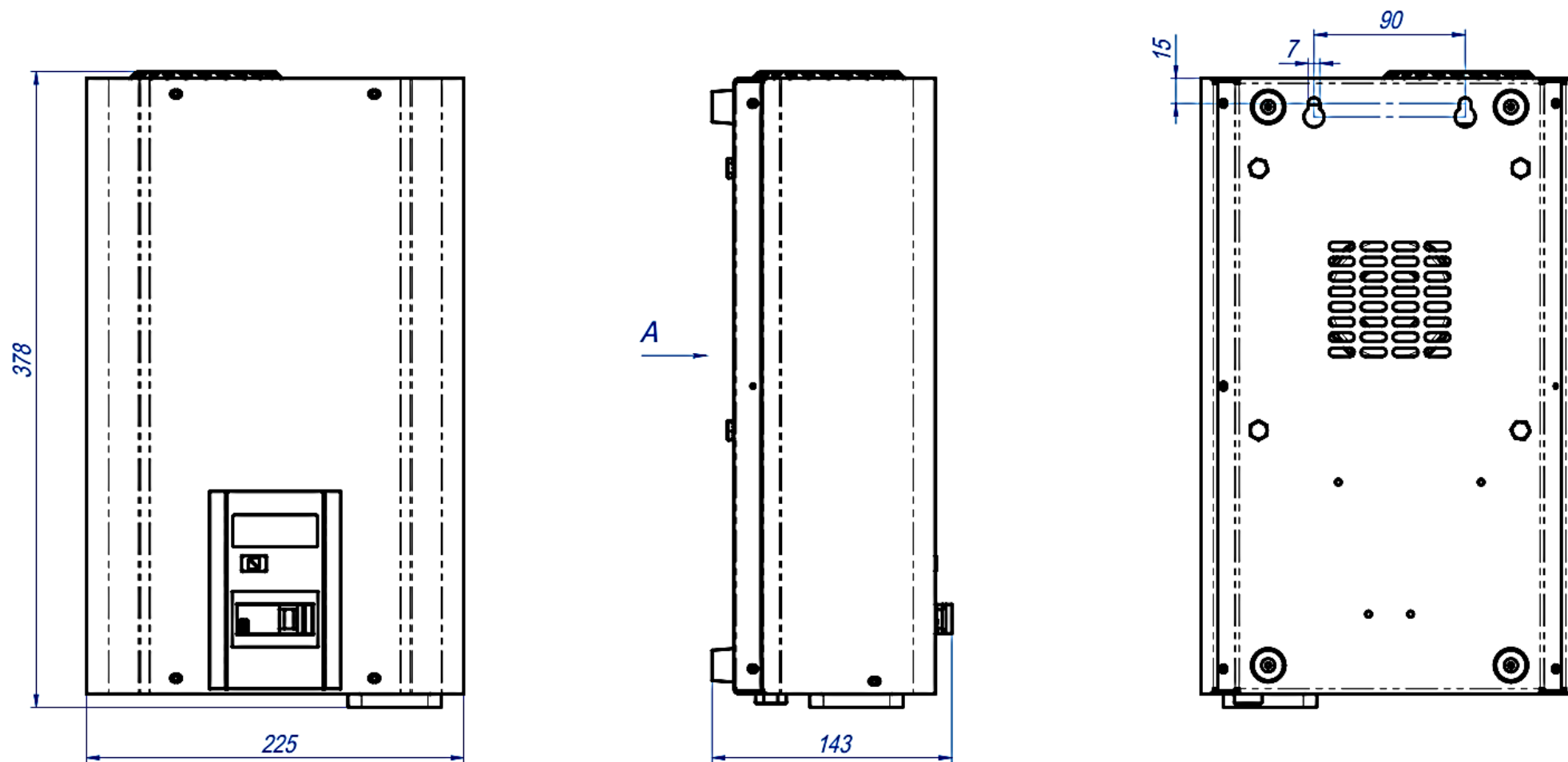
Габаритные и установочные размеры стабилизаторов ГИБРИД на 10- 16А
