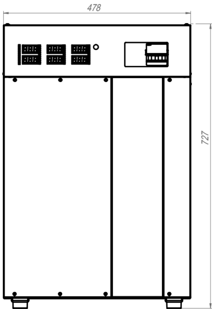
Габаритные размеры стабилизаторов Герц на 25-63А
