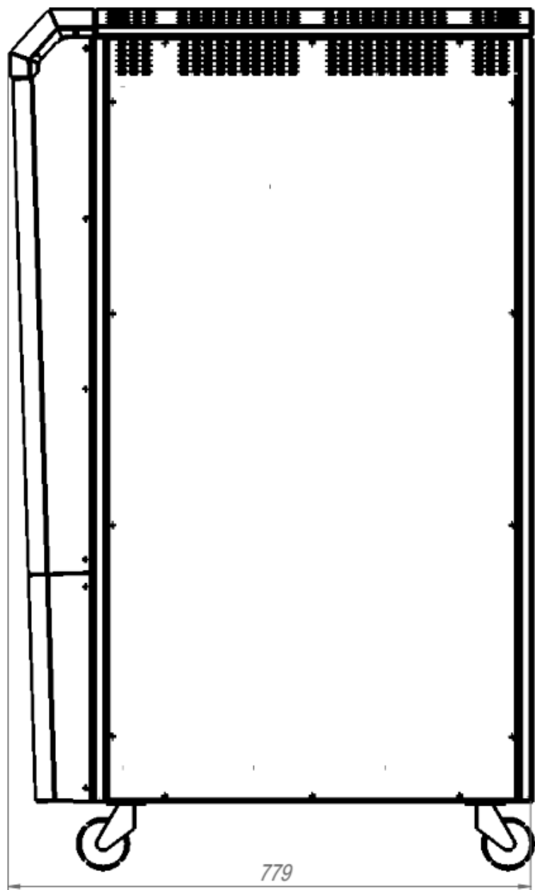
Габаритные размеры стабилизаторов Герц-ПРО на 100-160А
