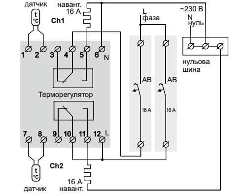
Схема 1. Підключення кожного каналу на окреме навантаження
