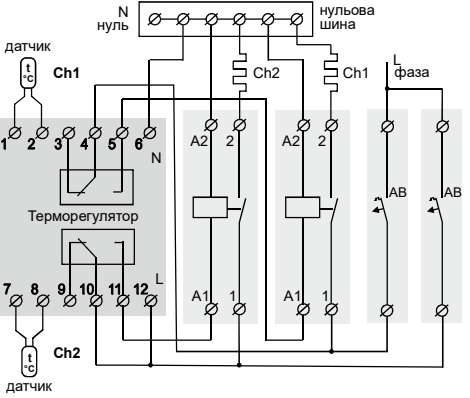
Схема 3. Використання контактора для збільшення комутованої потужності каналу
