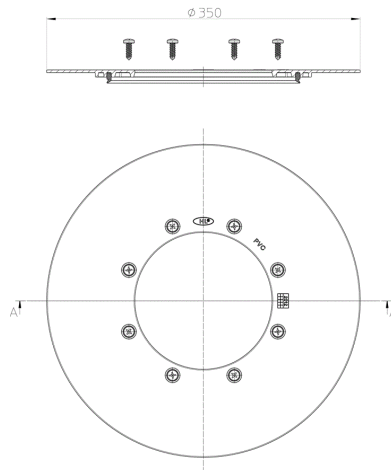
Schnitt A-A
