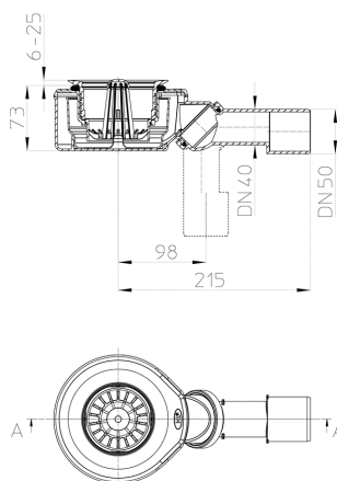
Schnitt A-A
