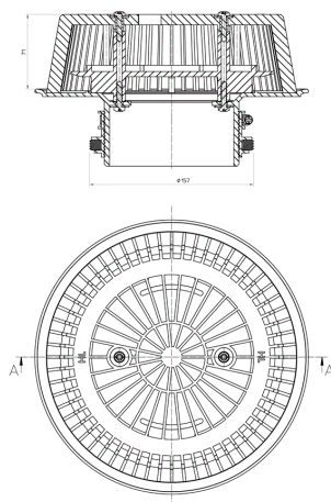
Schnitt A-A
