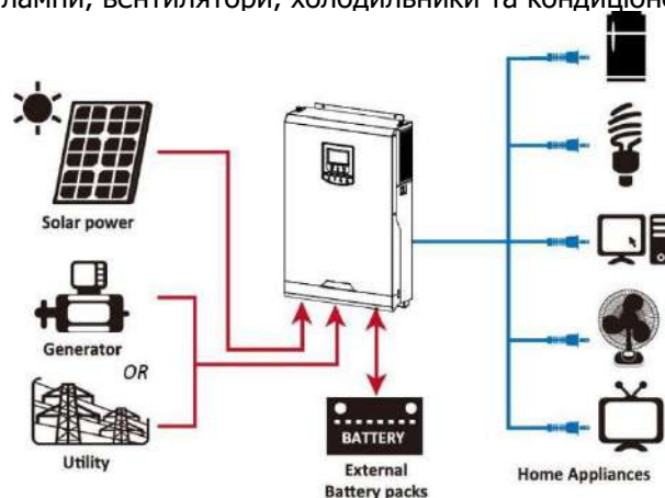
Рисунок 1. Гібридна енергосистема
