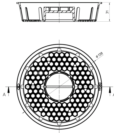
Schnitt A-A
