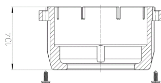
Schnitt A-A
