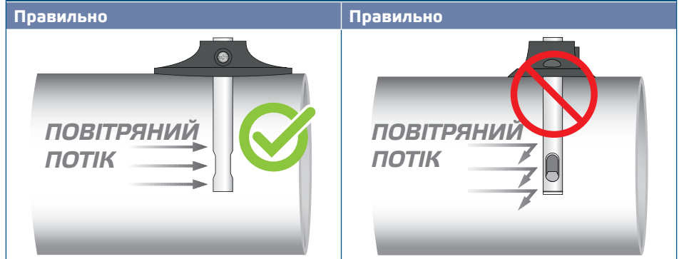
Мал. 2 Монтажне положення
