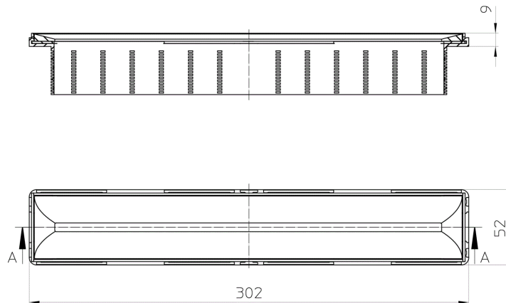
Schnitt A-A
