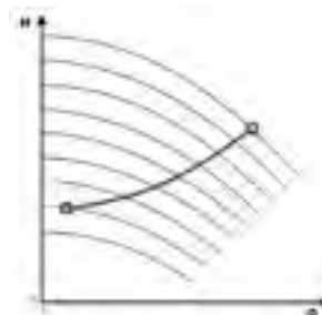
Регулировка по заданной кривой
