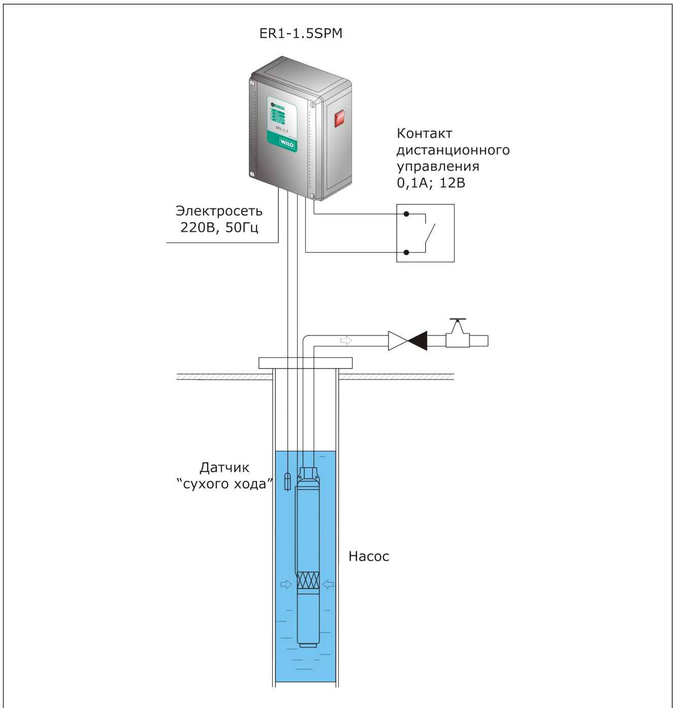
Рис.2 - Управление скважинным (погружным) насосом
