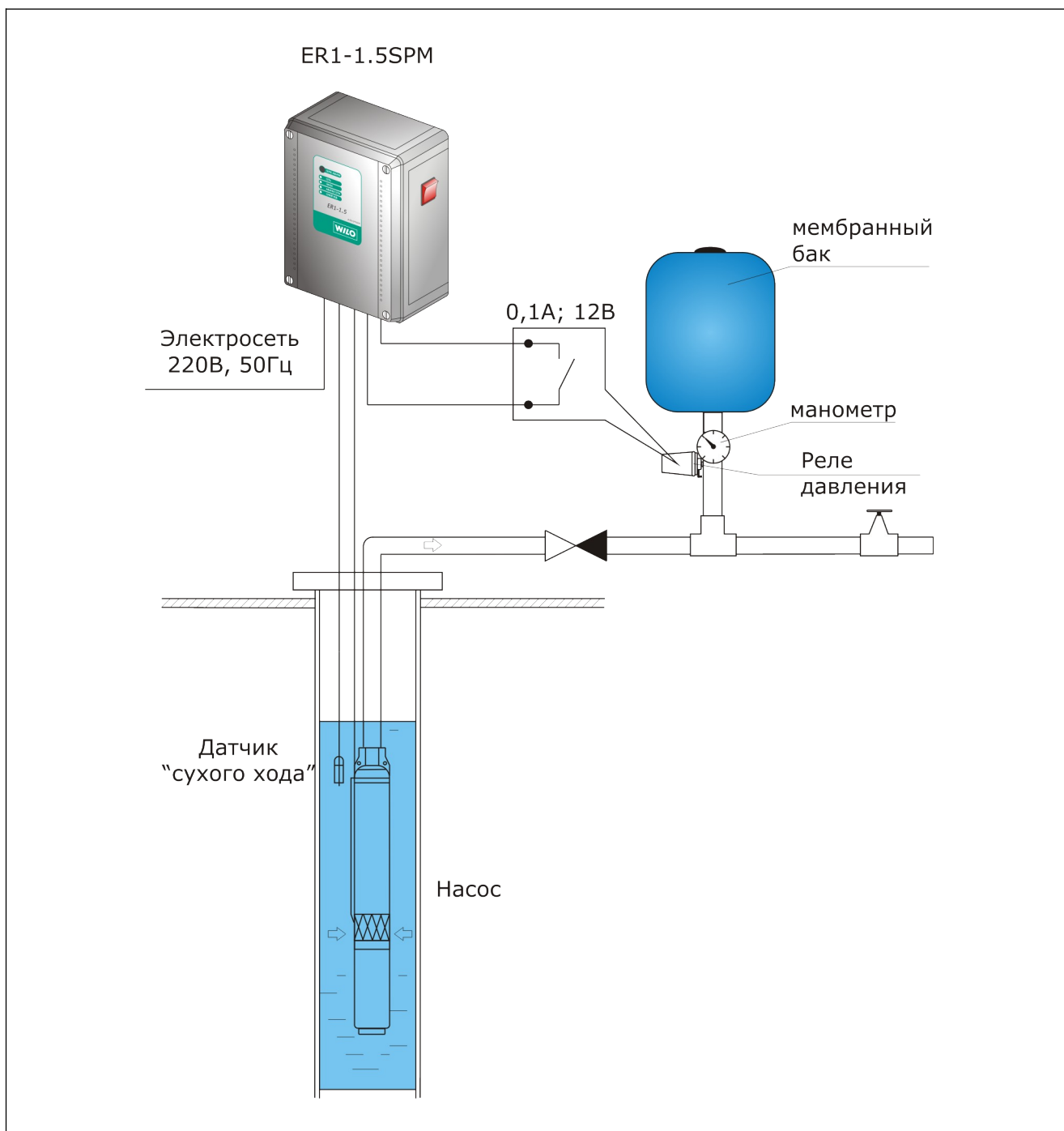
Рис.3 - Управление скважинным (погружным) насосом в системе повышения давления
