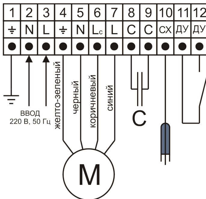
Подключение однофазного насоса без встроенного конденсатора
