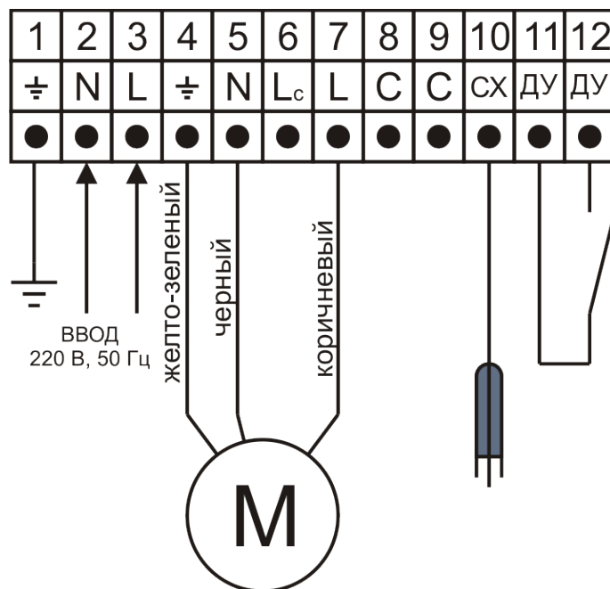
Подключение однофазного насоса со встроенным конденсатором
