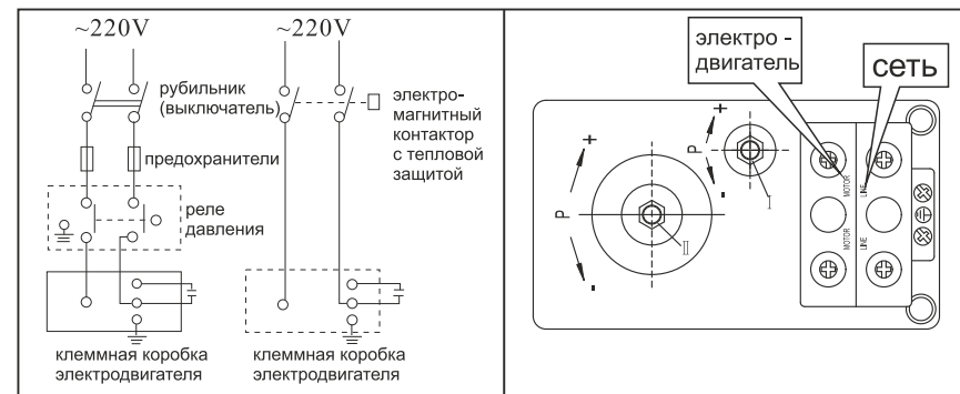
электрическая схема подключения насоса
