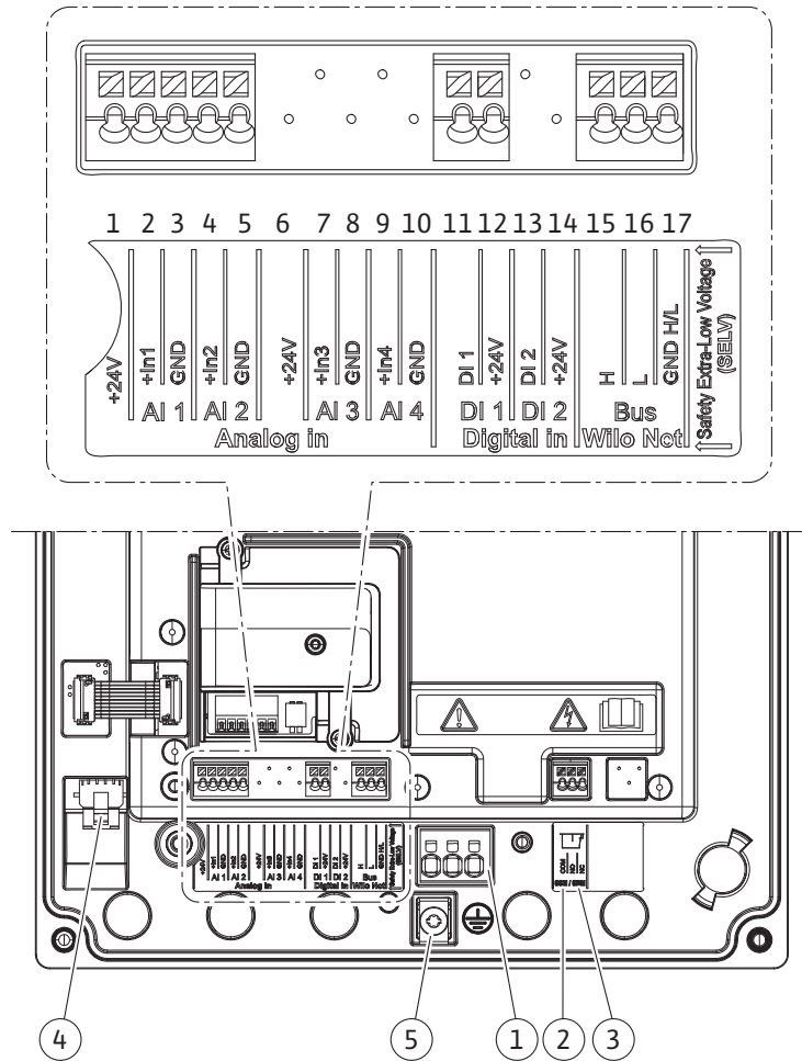
Fig. 9: Огляд клем у модулі
