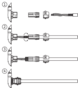
Fig. 15: Кабельний екран
