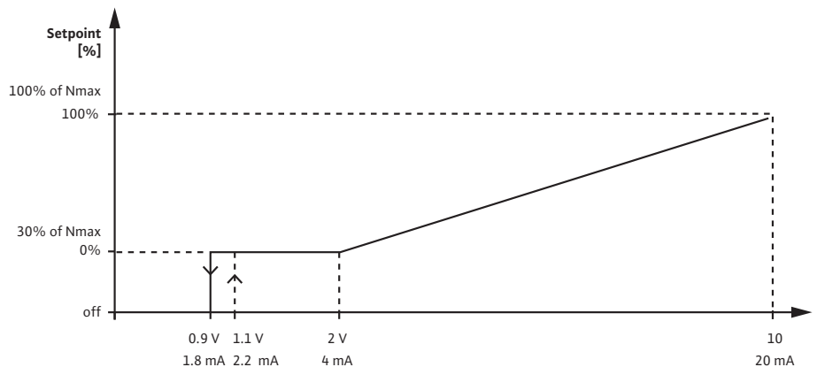
Fig. 25: Вхід заданого значення 0 – 10 В або 0 – 20 мА
