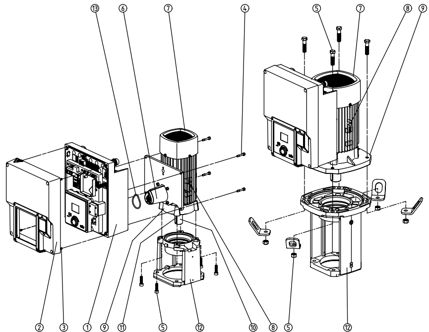
Fig. 1: Основні компоненти
