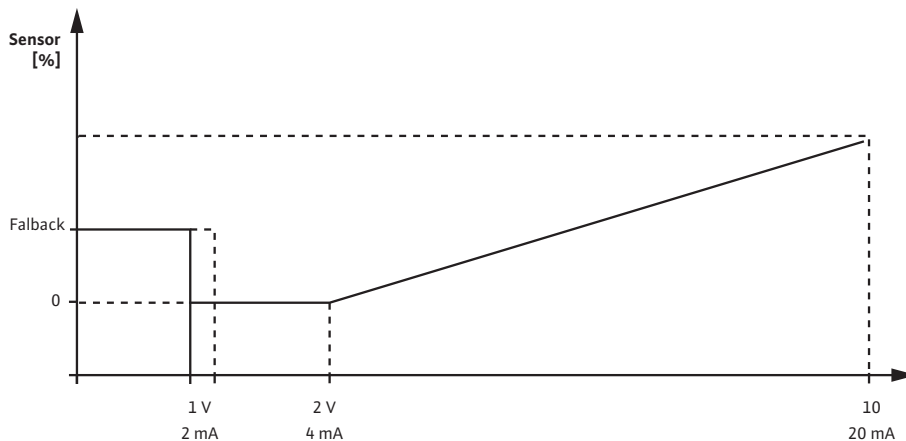
Fig. 28: Вхід давача 0 – 10 В або 0 – 20 мА
