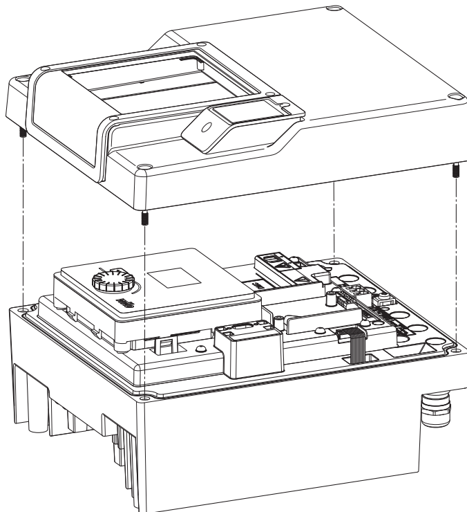
Fig. 31: Відкривання кришки електронного модуля
