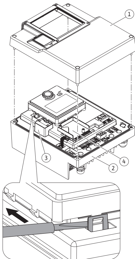
Fig. 16: Електронний модуль
