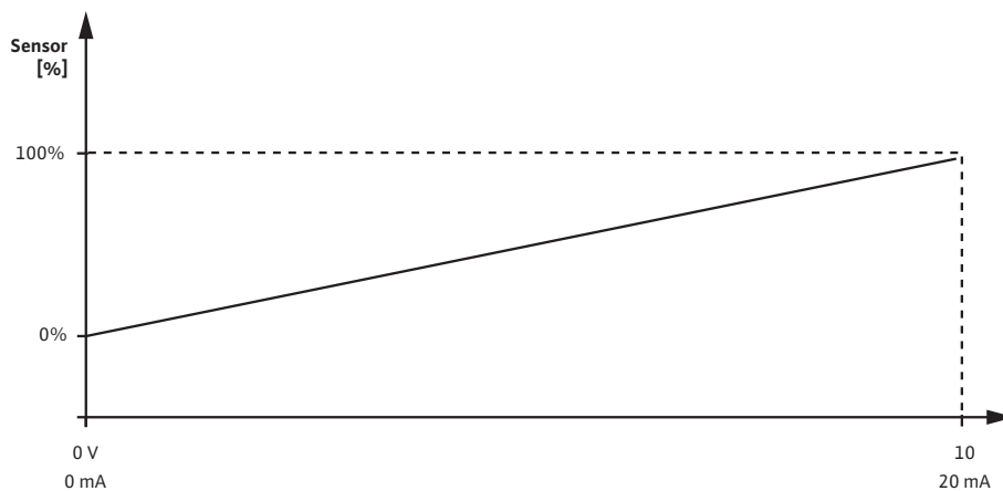
Fig. 27: Вхід давача 0 – 10 В або 0 – 20 мА
