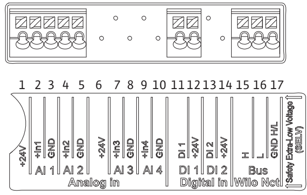
Fig. 10: Клеми для аналогових входів, цифрових входів і Wilo Net. Wilo Net AI3, AI4 і DI2 не зайняті.
