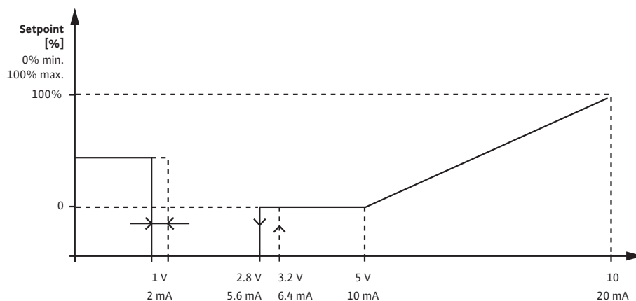
Fig. 26: Вхід заданого значення 2 – 10 В або 4 – 20 мА
