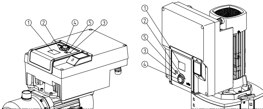
Fig. 18: Органи керування
