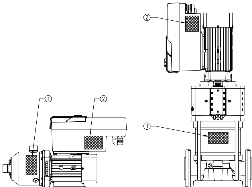
Fig. 3: Заводські таблички
