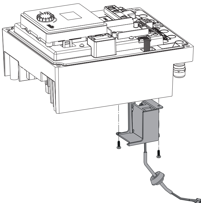
Fig. 34: Зняття вентилятора модуля разом із кабелем і гумовим ущільненням
