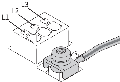
Fig. 11: Головне під'єднання заземлення
