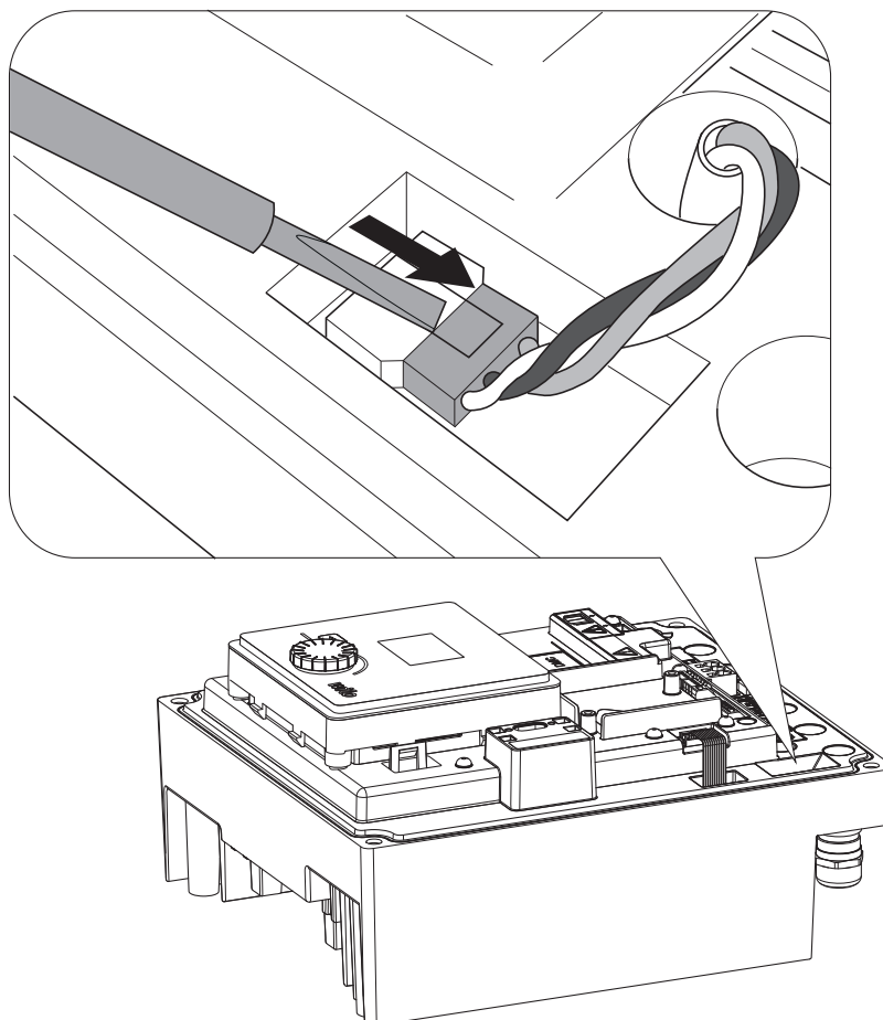
Fig. 32: Від'єднання під'єднувального кабелю вентилятора модуля
