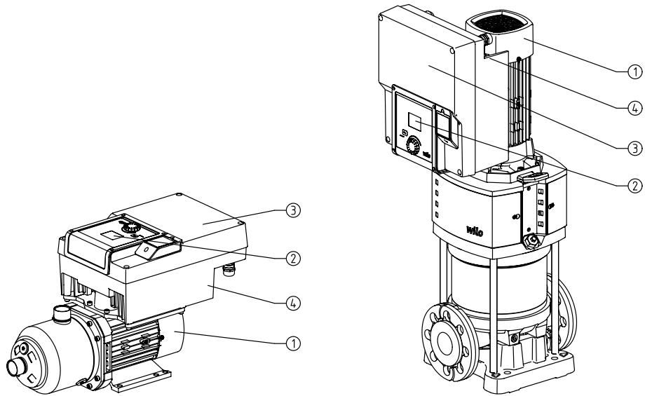
Fig. 2: Огляд привода
