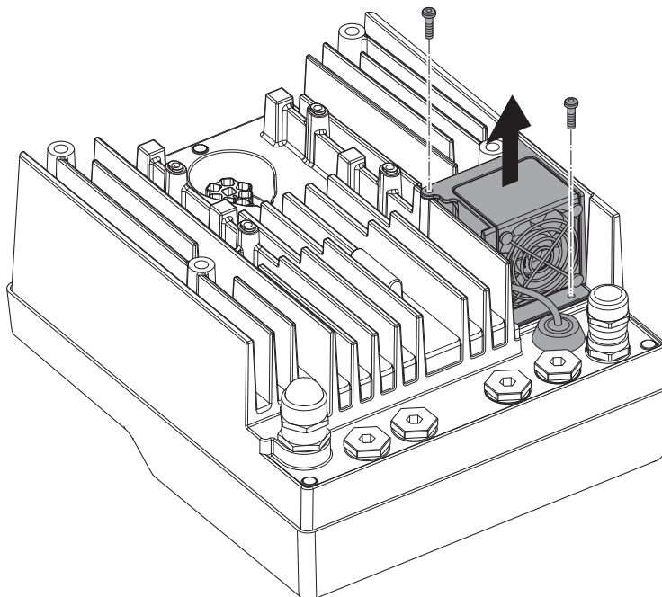
Fig. 33: Демонтаж вентилятора модуля
