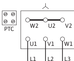
Fig. 11: Схема «зірка»
