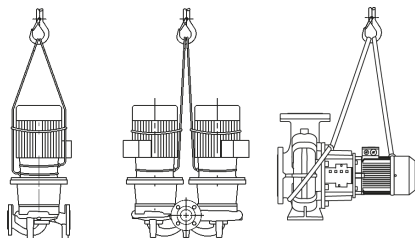
Fig. 1: Транспортування насоса
