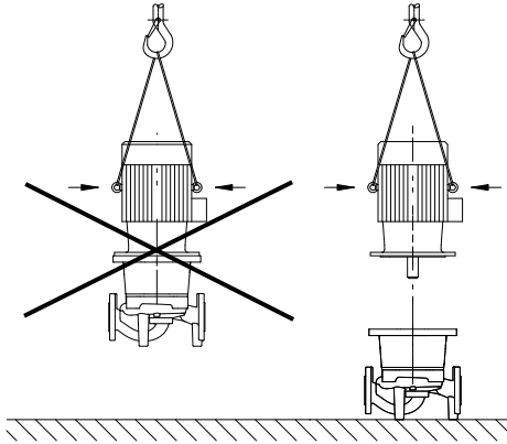
Fig. 2: Транспортування двигуна
