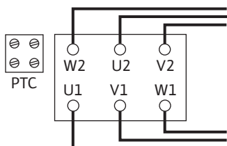
Fig. 12: Схема «трикутник»
