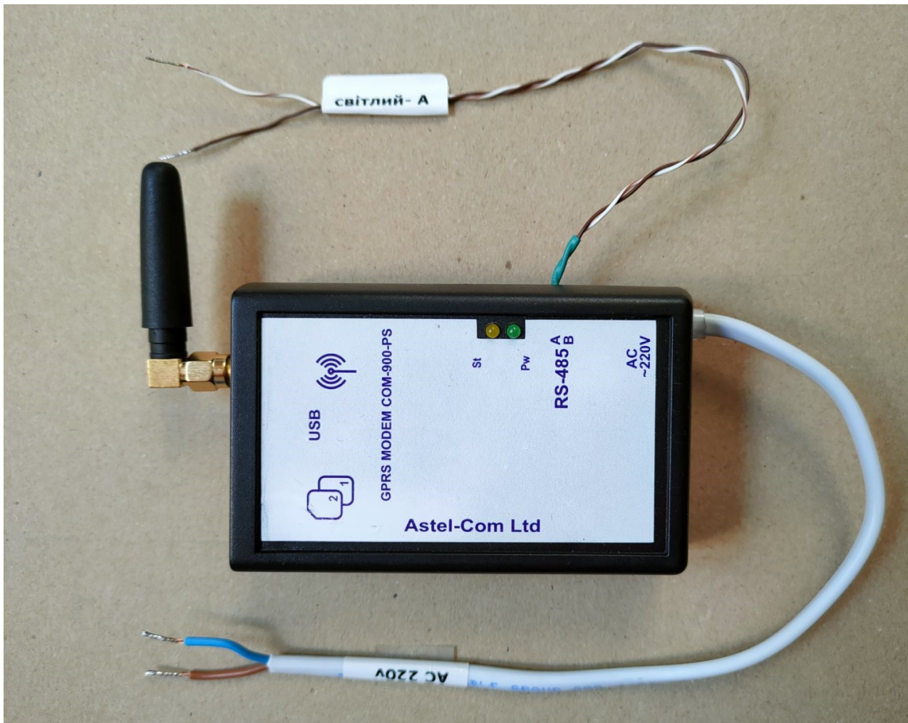
Мал. 1 Загальний вид модему COM-900-PSG rev.A.
