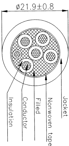
SEC A-A
