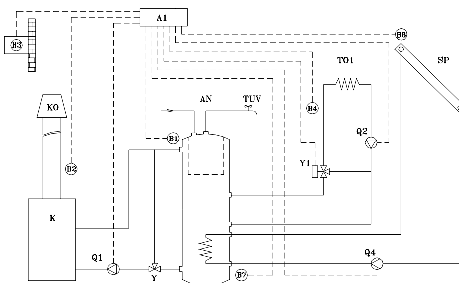
Рис. 7 Рекомендуемые (принципиальные) схемы подключения котла к отопительной системе.
