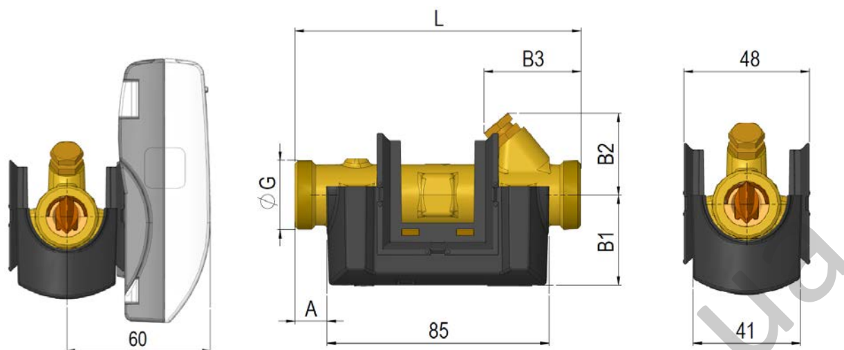
Рис. 5: Преобразователь расхода с резьбовым соединением G¾ и G1
