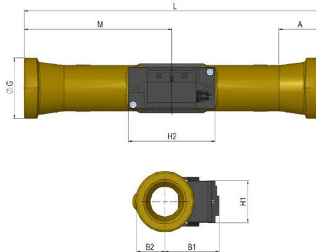
Рис. 6: Преобразователь расхода с резьбовым соединением G5/4 и G2
