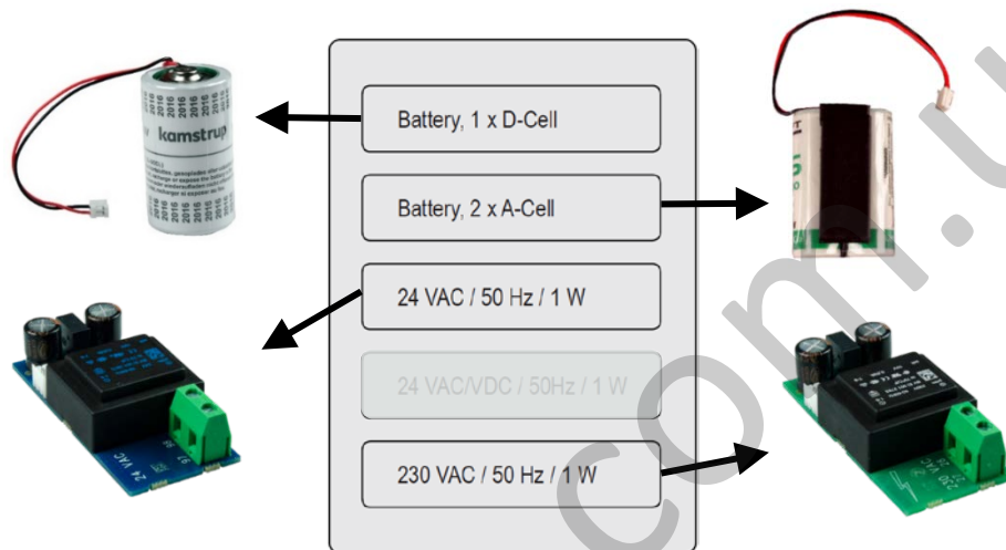
Figur 13 - Выбор наклейки для устанавливаемого модуля питания
