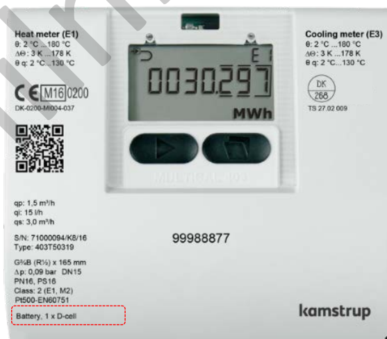
Figur 14 - Место нанесения наклейки на MULTICAL® 403
