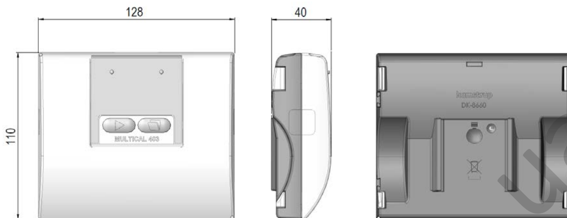
Рис. 2: Механические размеры вычислителя
