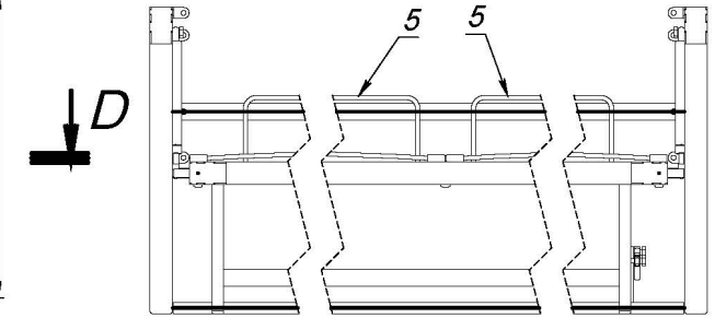
E-E (1 : 5)
