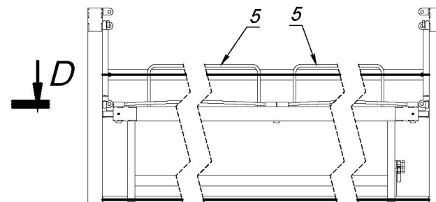
E-E (1 : 5)
