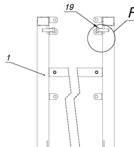
E-E (1 : 5)
