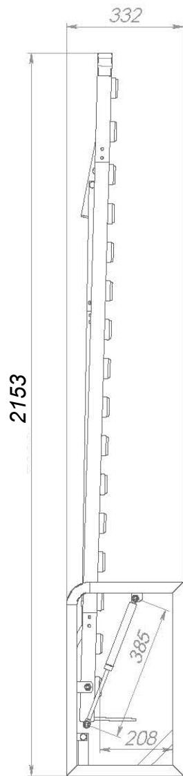
Вертикальная 900x2000 (крепление к стене или полу)
