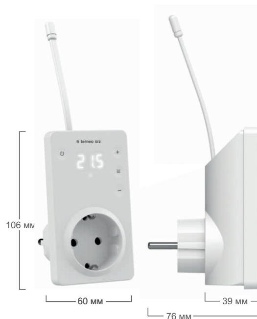
Рисунок 1. Габаритні розміри terneo srz
