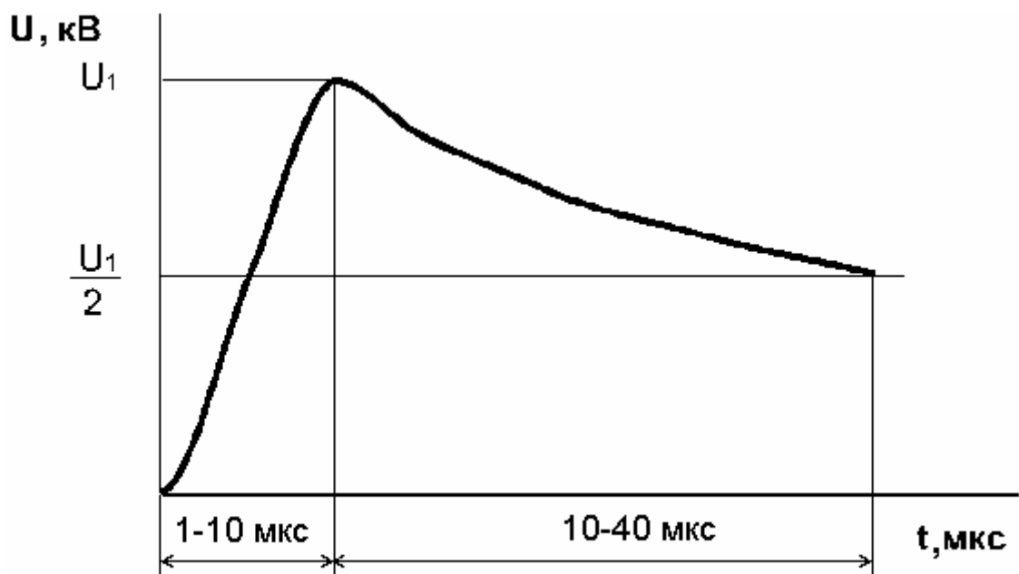
Рисунок Д.4 - Форма грозовых импульсов, характерная для точек присоединения б, е, ж на рисунке Д.1.
