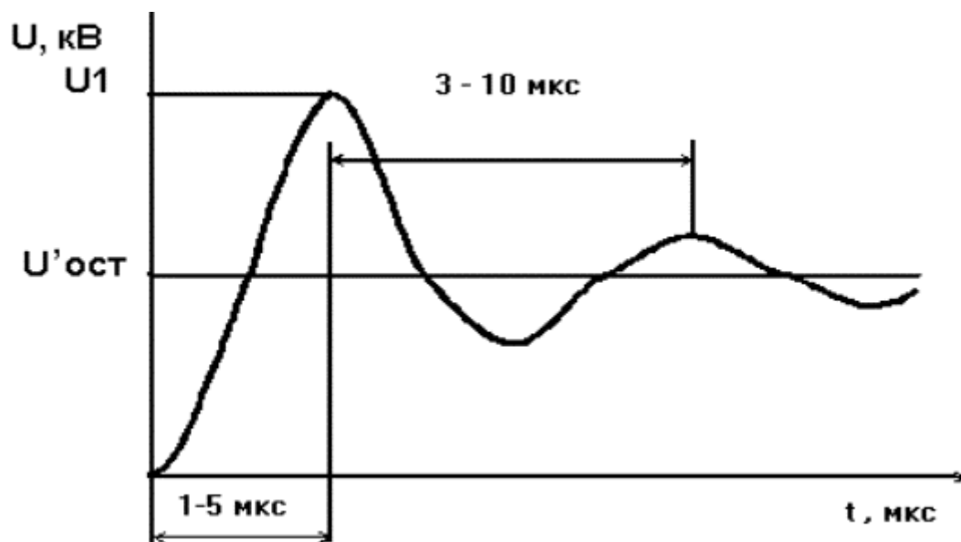
Рисунок Д.2 - Форма грозových импульсов, характерная для точек присоединения а, в, г, д на рисунке Д.1.
