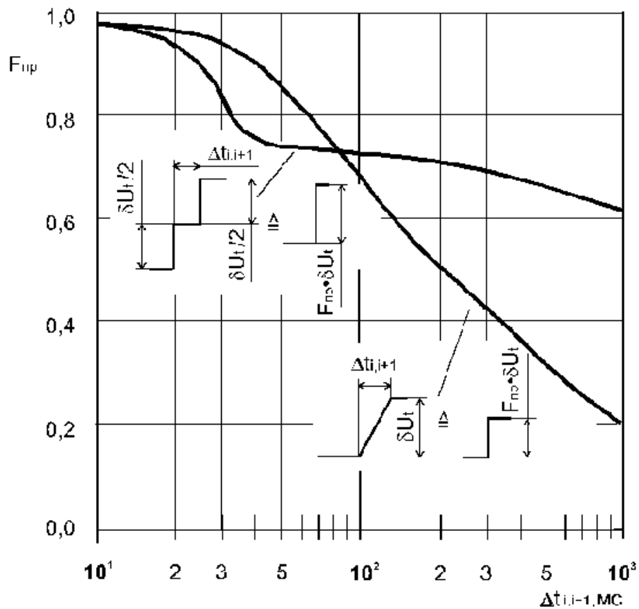
Рисунок В.1 - Коэффициент приведения F_{пр} для периодических колебаний напряжения, имеющих двухступенчатую и пилообразную форму
