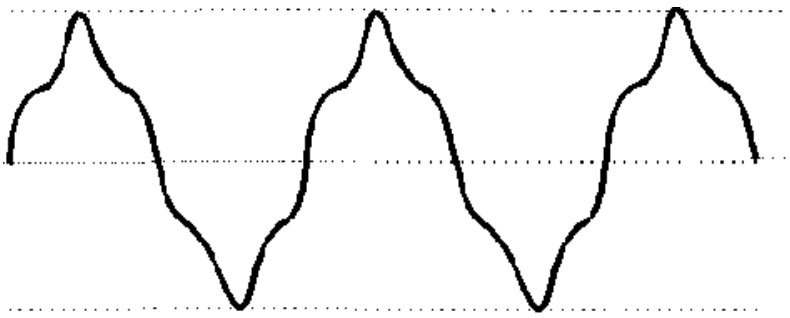
Рисунок А.2 - Несинусоидальность напряжения
