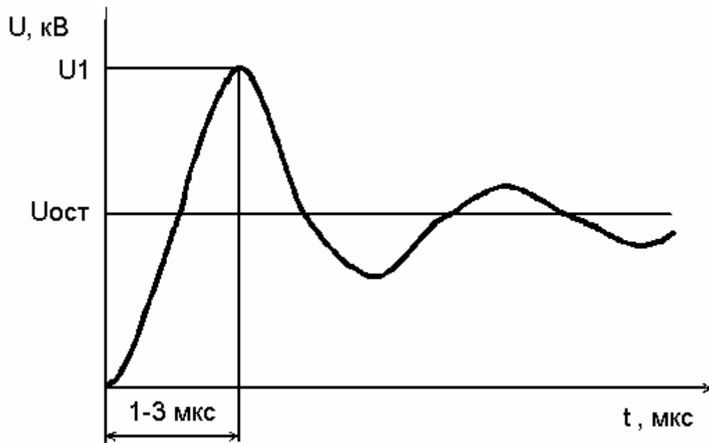
Рисунок Д.2 - Форма грозových импульсов, характерная для точек присоединения а, в, г, д на рисунке Д.1.
