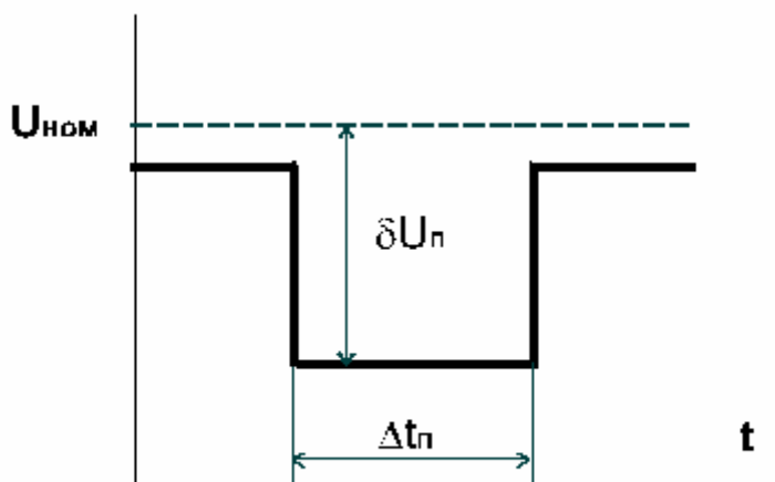
Рисунок Б.2 - Провал напряжения
