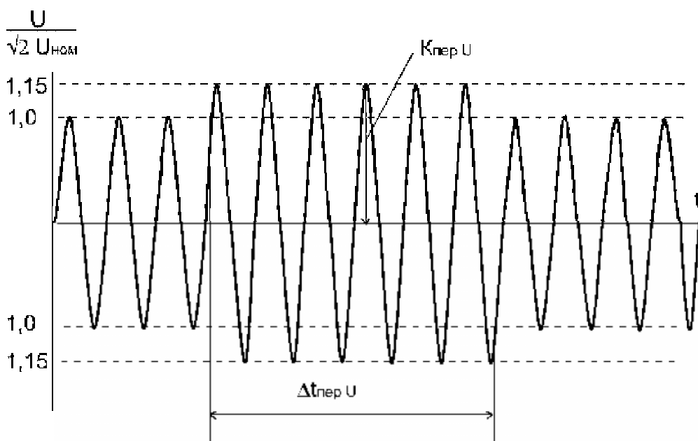
Рисунок Б.4 - Временное перенапряжение
