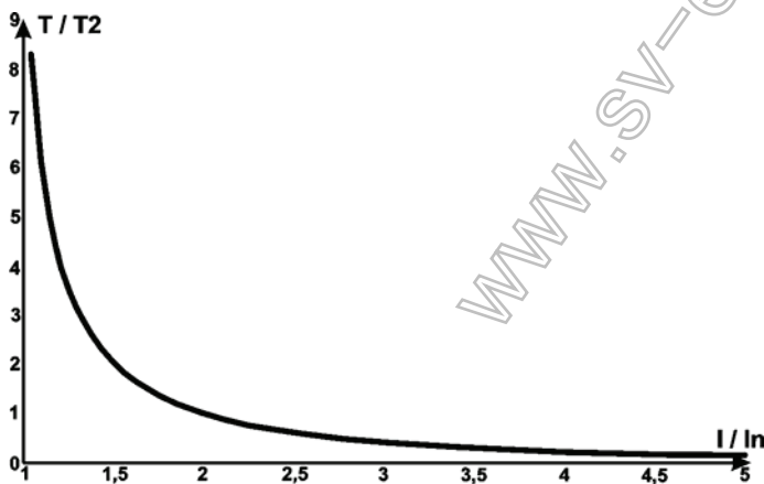
Рисунок 7 – Токо-временная характеристика
