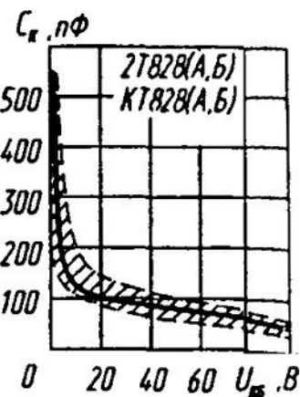
Зона возможных положений зависимости емкости коллекторного перехода от напряжения коллектор—база
