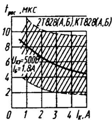
Зона возможных положений зависимости времени рассасывания от тока коллектора
