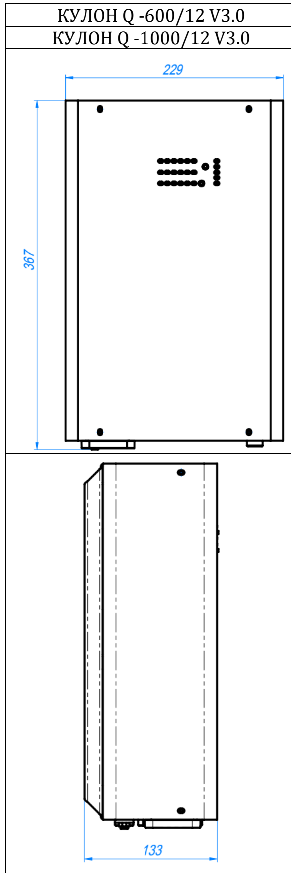
Рисунок 6. Габаритные размеры ИБП
