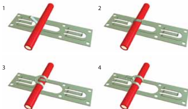
Рисунок 12.1. Поэтапное крепление кабеля на ленту DEVIfast™
