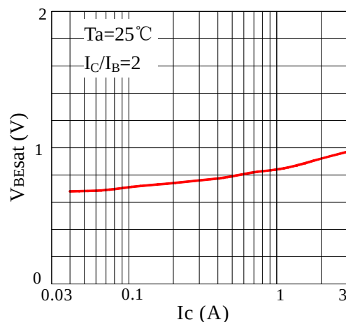
Fig6 VBESat-Ic
