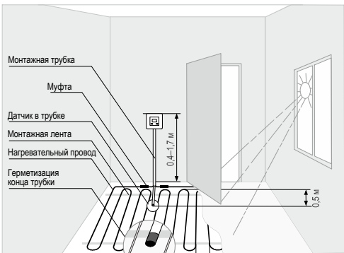
Рисунок 1. Монтаж терморегулятора и теплого пола
