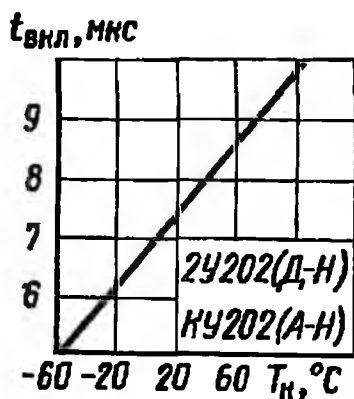
Зависимость времени включения от температуры корпуса
