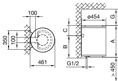
Рис. 1: Монтаж на стену в вертикальном положении
