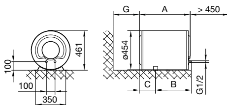
Fig. 2: Montarea orizontală pe podea
