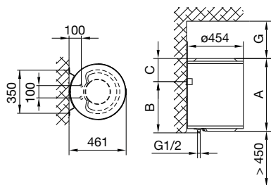
Fig. 1: Instalarea boilerului pe perete în poziție verticală
