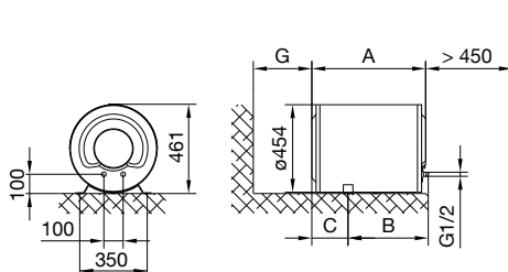
2 Сурет: Еденге көлденеңінен орнату
