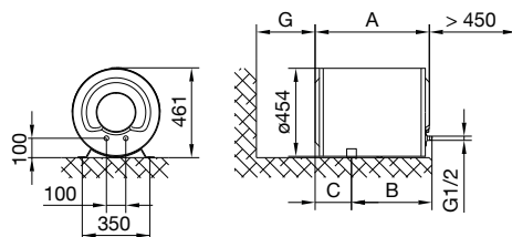
Sl. 2: Vodoravno montiranje na pod
