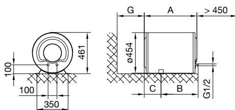
Рис. 2: Горизонтальная установка на полу
