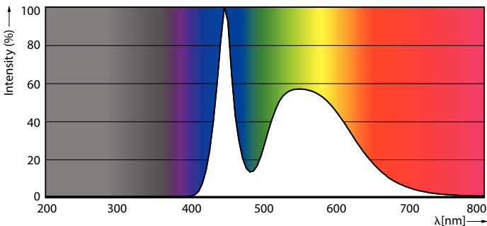
LEDtube ECO RCA 18W G13 1650lm 765-POC
