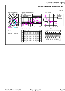
LEDtube Ecofit 8W G13 840 24D ND
